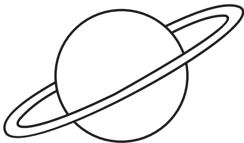
URANUS
