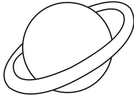
SATURNUS
