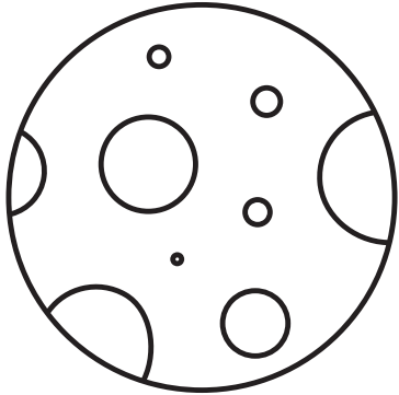
MOON
